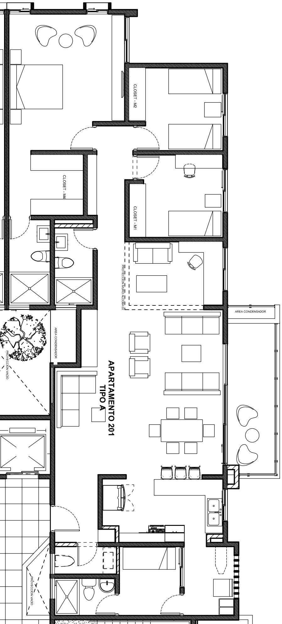
1 PLANTA GENERAL APTOS TIPO A PISO TIPO
