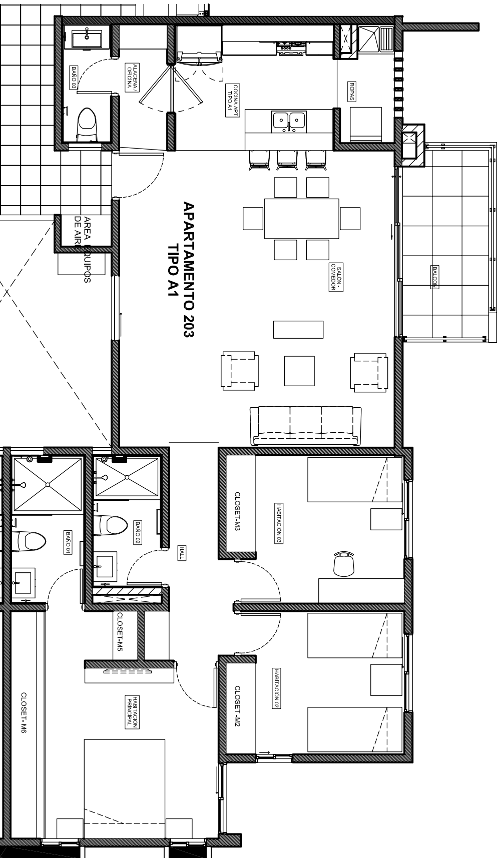
1 PLANTA APTO TIPO A1-A1' PISO 2
