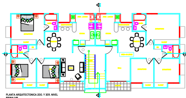
PLANTA ARQUITECTONICA 2DO. Y 3ER. NIVEL ESCALA 1:50
